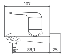
IN02 M.R.P. ₹ : 1545/- Bib Cock
