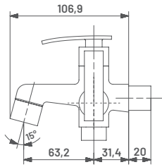
BR08 M.R.P. ₹ : 2060/- 2 Way Bib Cock
